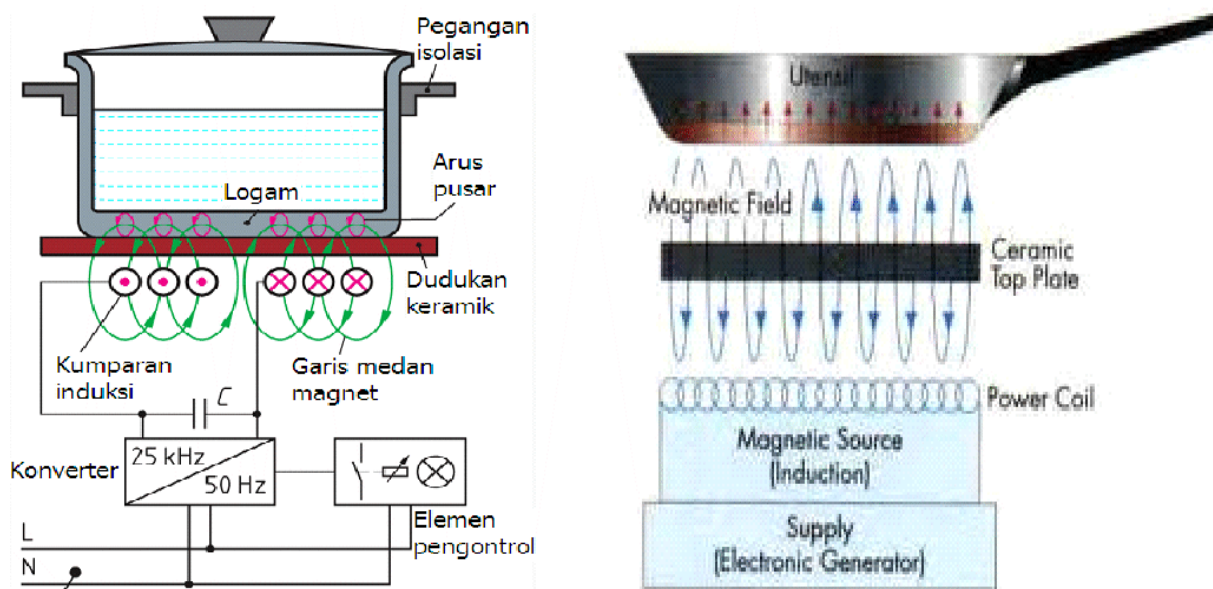
Gambar 1. Prinsip Kerja Kompor Induksi
