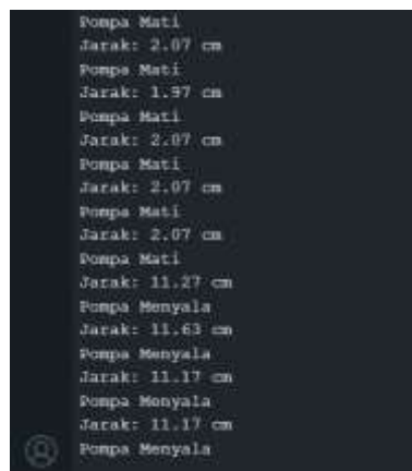
Gambar 4. Respon Pompa Air pada Serial Monitor Arduino
